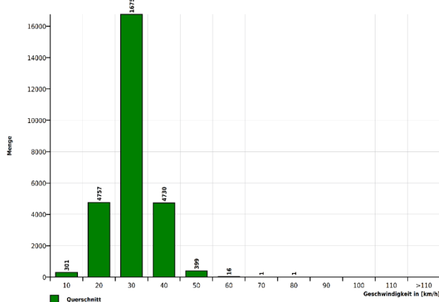
Geschwindigkeits-Histogramm
